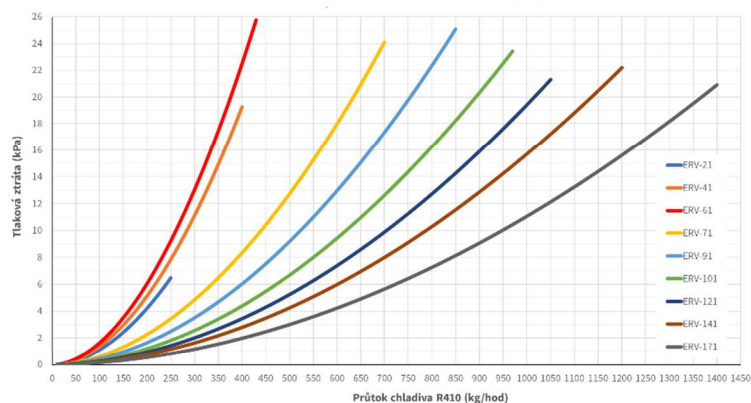
Tlaková ztráta výměníku ERV chladič okruh (kPa)
