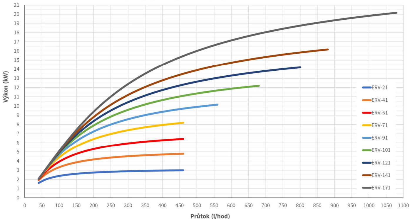
Tepelný výkon výměníků (kW) Teplota vstupní vody 13,8 °C, Teplota par chladiva na vstupu = 58,0 °C
