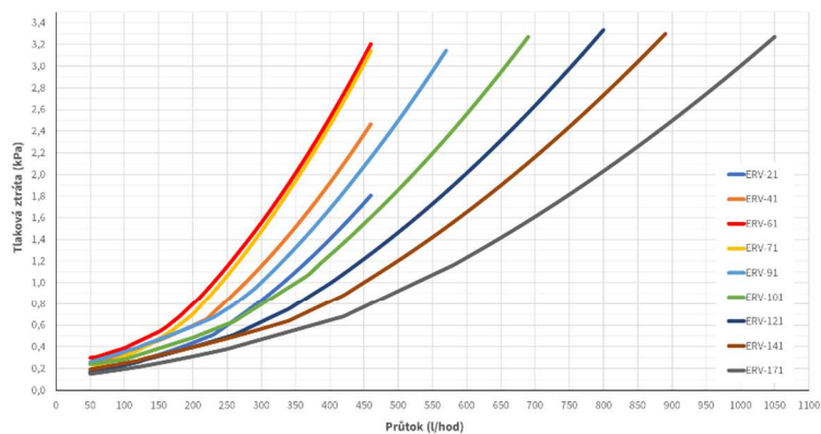
Tlaková ztráta výměníku ERV vodní okruh (kPa)
